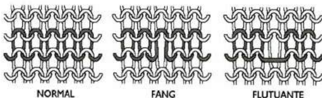
Figura 1. Representación gráfica del punto de mallas cogidas
